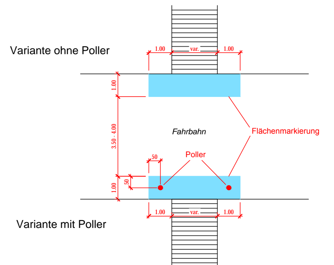
Detail Fussweganschluss Masstab 1:100
